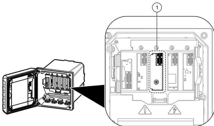
図 2 EtherNet/IP モジュールスロット
