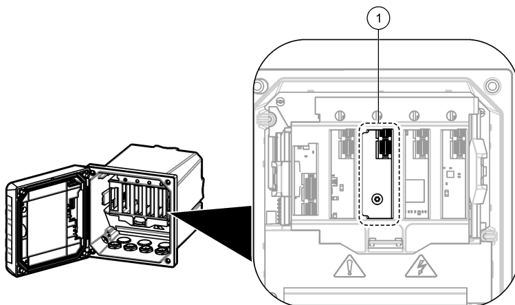
Figura 2 Slot do módulo EtherNet/IP
