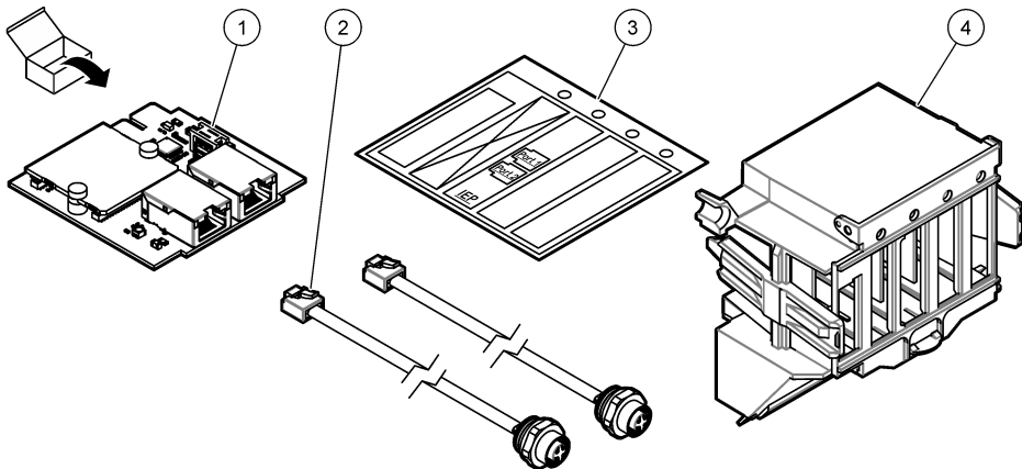
รูปที่ 1 ส่วนประกอบของผลิตภัณฑ์
