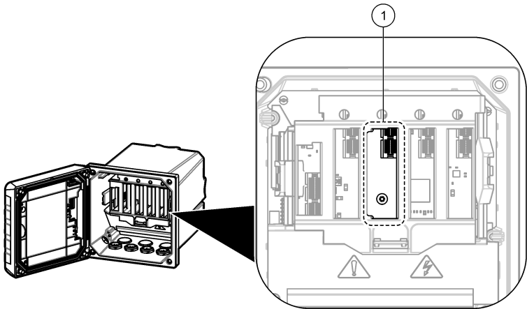
1 สล็อตโมดูล EtherNet/IP
