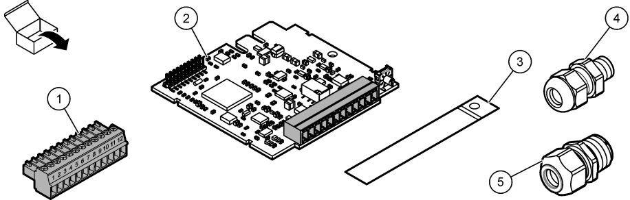
الشكل 1 مكونات المنتج
