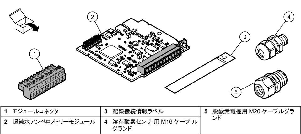
図 1 製品構成部品
