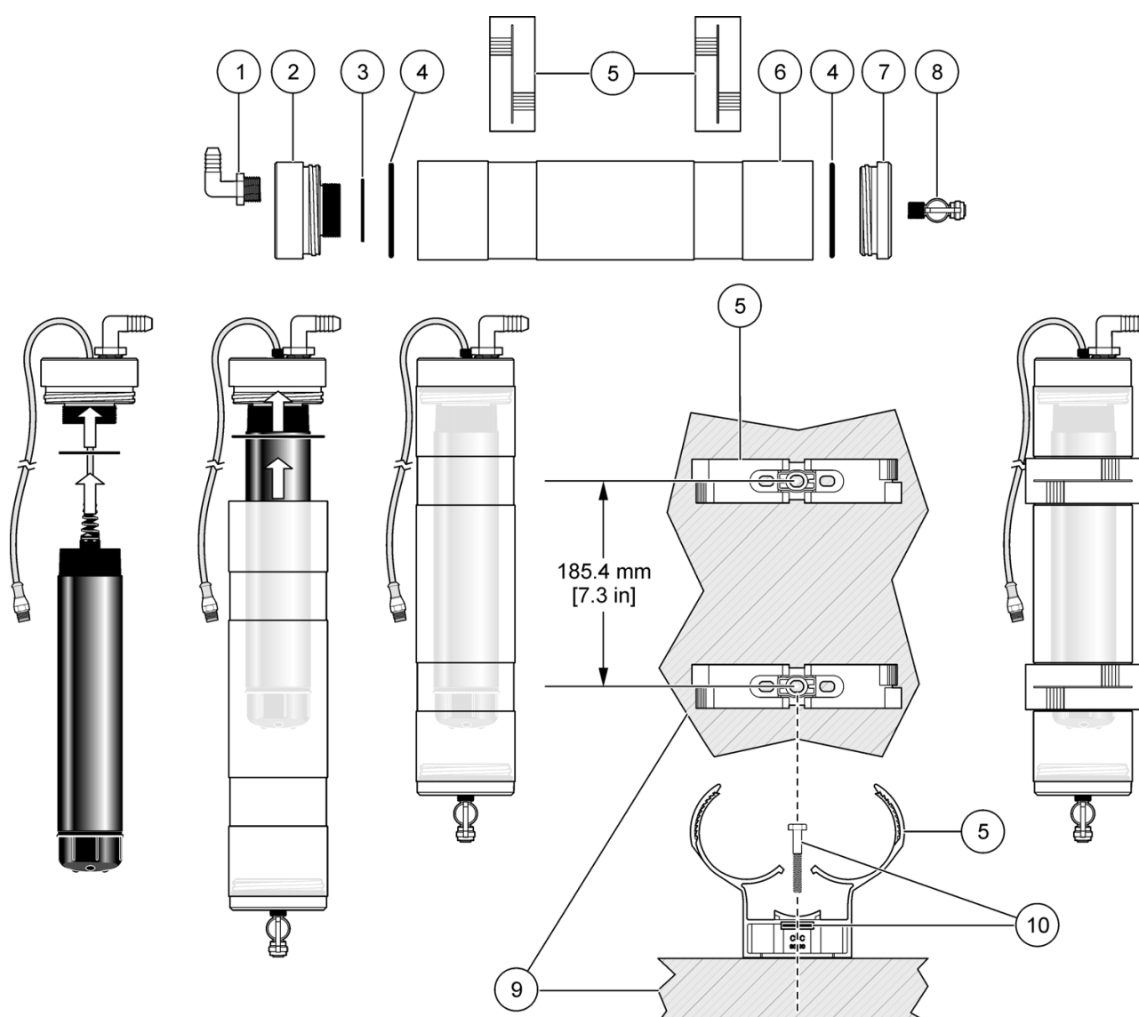
figur 1 Installation av LDO flödescell och givare
